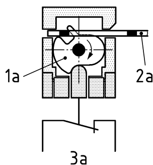
a) bewegliche trennende Schutzeinrichtung geschlossen
