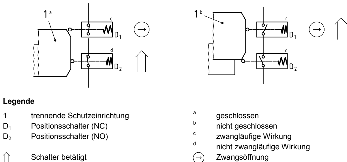
Bild 13 — Vermeidung von Ausfällen gemeinsamer Ursache von zwei mechanisch betätigten Positionsschaltern durch eine verbundene zwangsläufige und nicht zwangsläufige Wirkung
