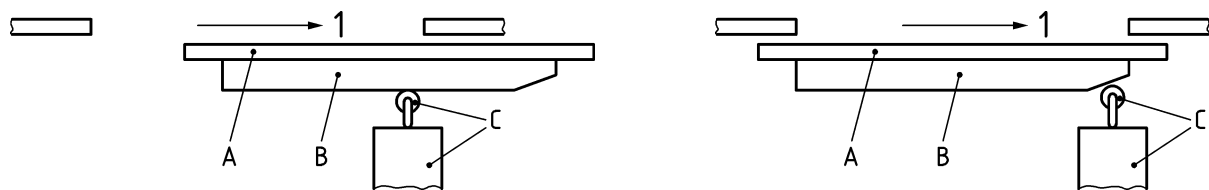
a) bewegliche trennende Schutzeinrichtung nicht geschlossen
