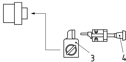
b) nicht betätigt mit erlaubtem Zugang
