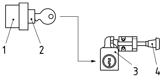
a) betätigt mit verwehrtm Zugang
