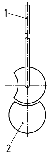
b) bewegliche trennende Schutzeinrichtung nicht geschlossen
