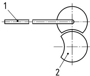
a) bewegliche trennende Schutzeinrichtung geschlossen
