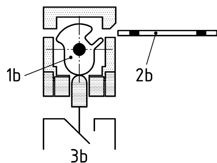
b) bewegliche trennende Schutzeinrichtung nicht geschlossen
